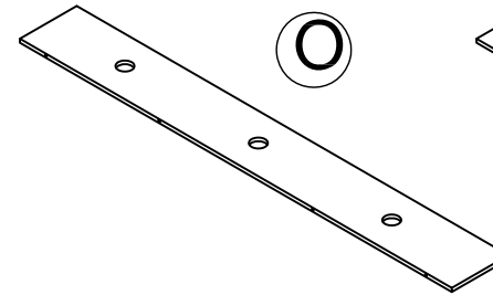
UPPER BACK PANEL Panel trasero superior PANNEAU ARRIÈRE SUPÉRIEUR T1781096050
