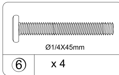
Bolt TSF1601
