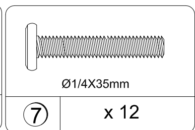
Bolt TSF1602
