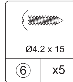
SCREW Tornillo VIS TEL4506
